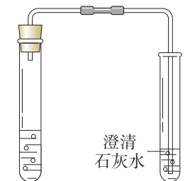
图 4-4 碳酸钠与盐酸反应的装置
