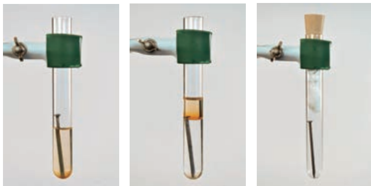
图 1-23 铁钉锈蚀条件的探究
