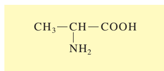
图 5-2 丙氨酸
