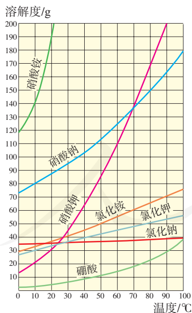
图2-12 几种固体物质的溶解度曲线
