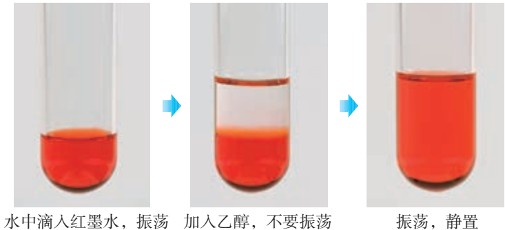
图2-4 乙醇能溶解在水中
