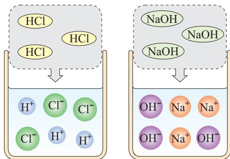
图3-10 \text{HCl} 和 \text{NaOH} 在水中解离出离子
