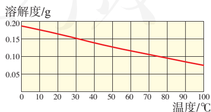
图2-13 氢氧化钙的溶解度曲线
