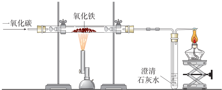
图 1-20 一氧化碳还原氧化铁
