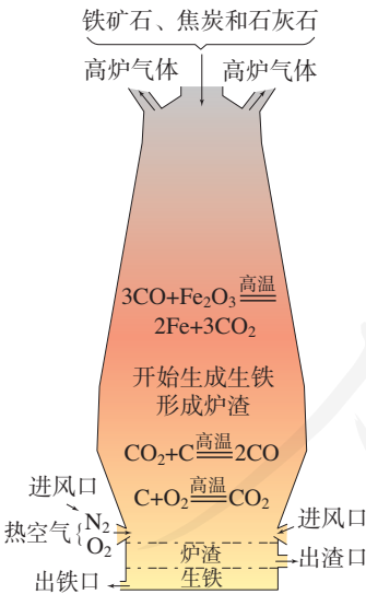
图 1-21 炼铁高炉及炉内化学反应过程示意图
