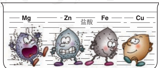
图1-12 金属与盐酸反应的比较
