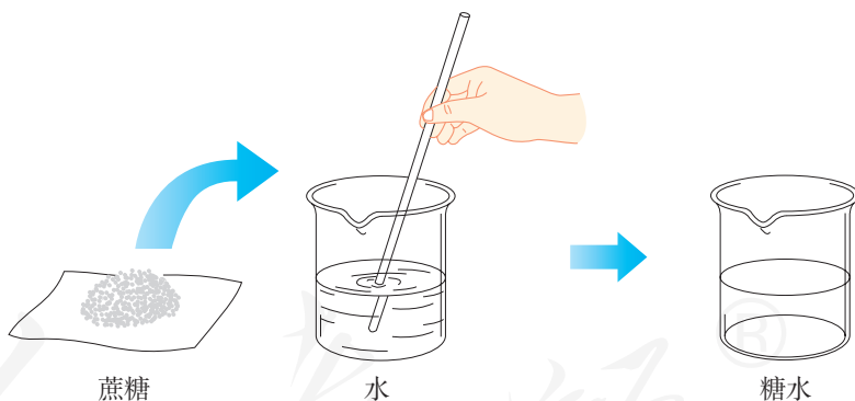
图2-2 蔗糖溶解
